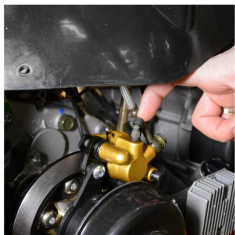
ВИНТ КЛАПАНА ВЫПУСКА ВОЗДУХА
