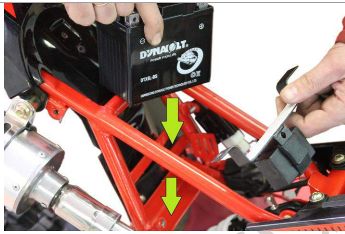
3.8.6. Снимите пластину крепления АКБ, открутив болт и установите АКБ на штатное место.
