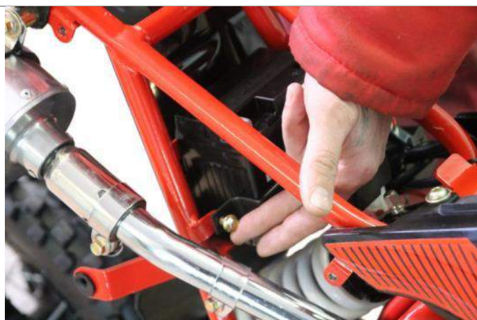
3.8.7. Установите пластину крепления АКБ и зафиксируйте болтом, который был выкручен ранее.
