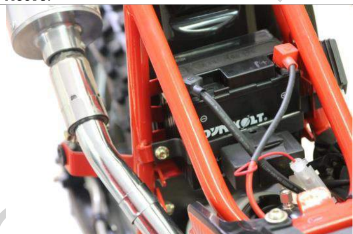
3.8.8. Установите клеммы согласно полярности, где красный это «+», черный соответственно «-».
