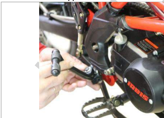
3.12.1 Установите кик-стартер на вал кик-стартера.
