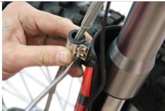
3.6.6 Зафиксируйте тормозной шланг хомутом, который находится на левом амортизаторе.
