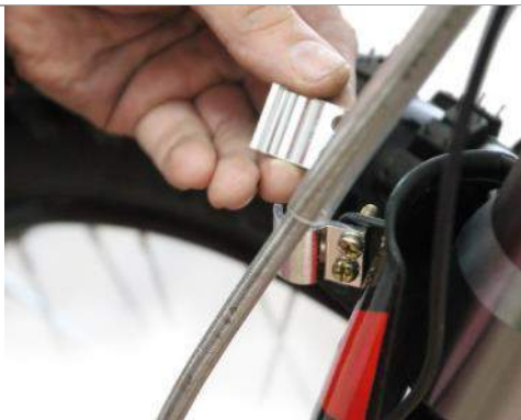
3.6.6 Зафиксируйте тормозной шланг хомутом, который находится на левом амортизаторе.
