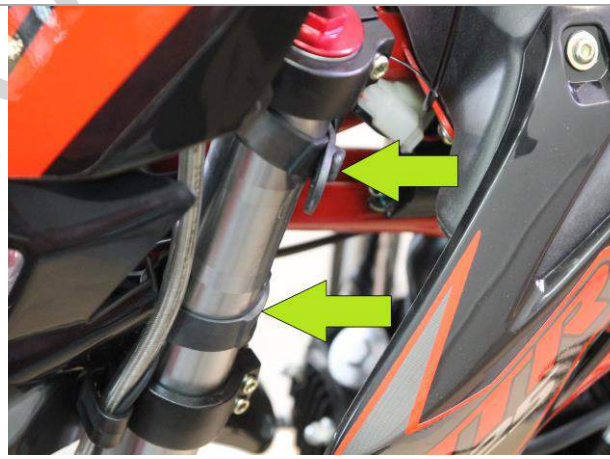
3.7.3. Зафиксируйте хомуты, которые находятся на фаре, к левой стойке амортизаторов и выровняйте фару.
